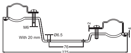
Collectors Assembling Clamps (1") Montage Klemmen für Kollektor (1")
